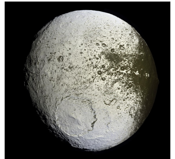
Iapetus
