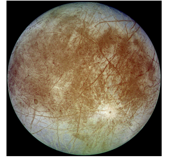
Europa
