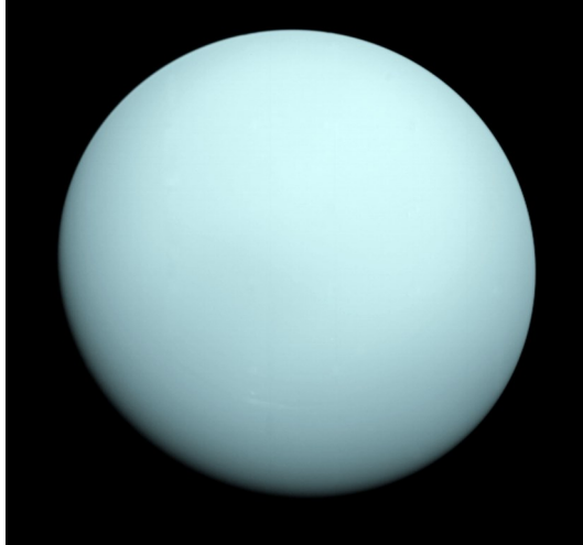
Uranus
