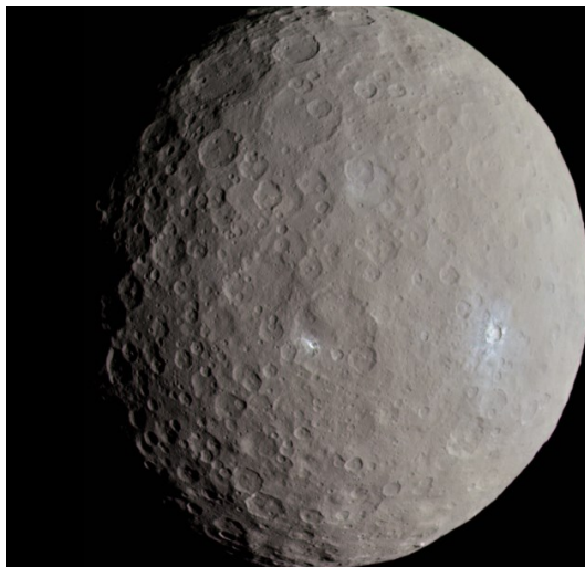
Ceres
